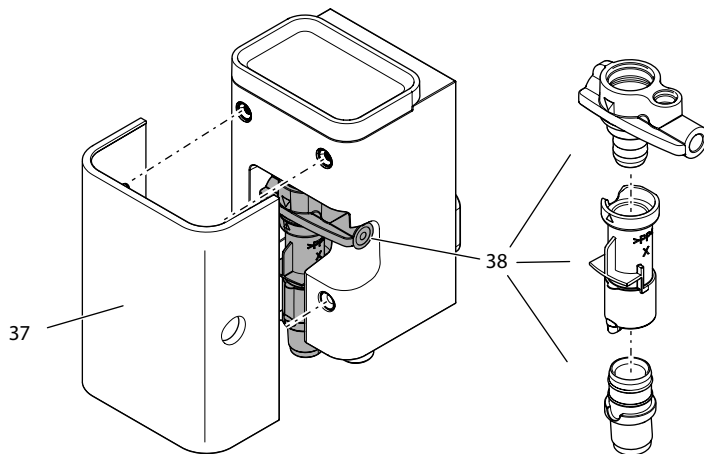
Bild 19: Demontera mjölkenheten
