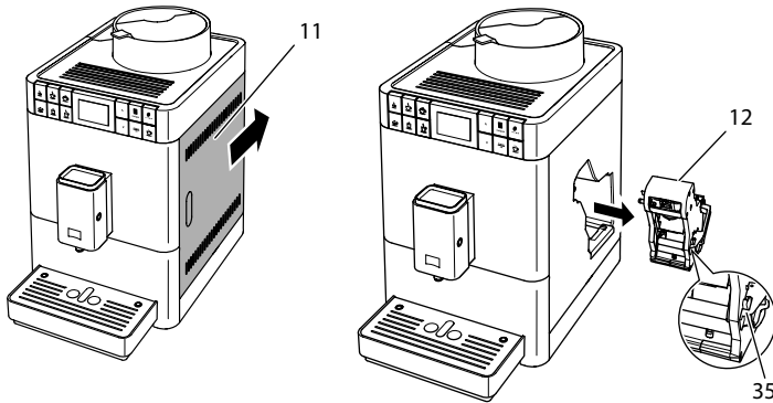
Fig. 17: Udtage brygheden
